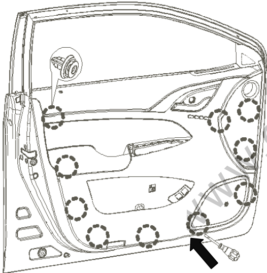
图1.9.7 门板拆卸
