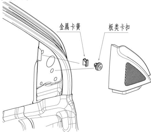
图1.9.11 角护板拆卸
