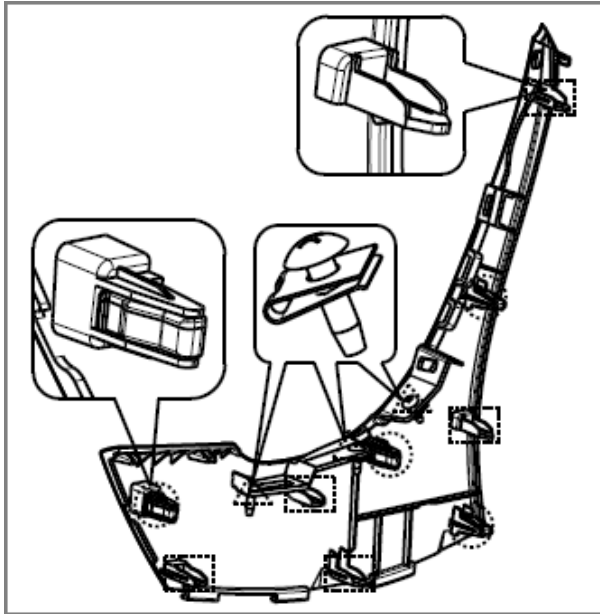
图 1.5.17 中控左护板
