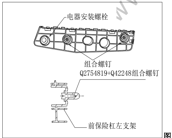
图 1.1.8 前保支架的拆卸
