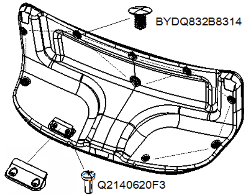
图 1. 15.4 行李箱盖护面 安装结构图
