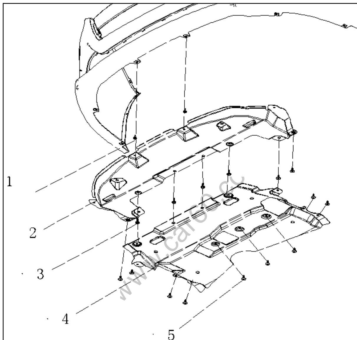
图 1.3.3 发动机下挡泥板的拆卸/安装
