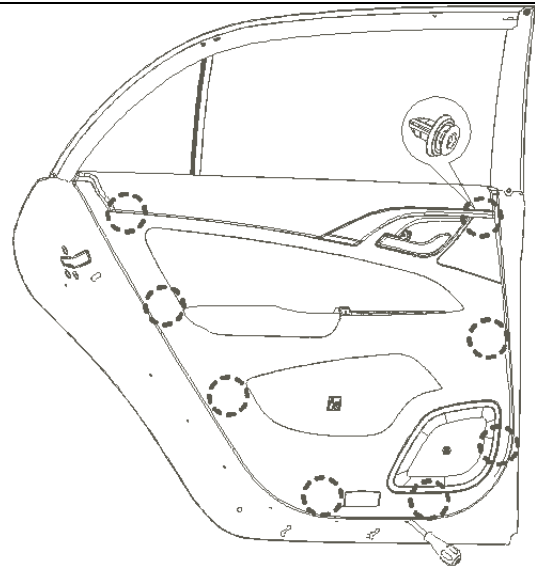
图1.9.18 门板拆卸
