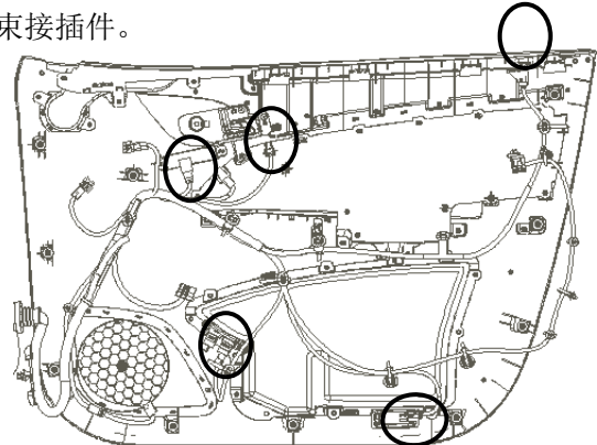
图1.9.10 线束拆卸
