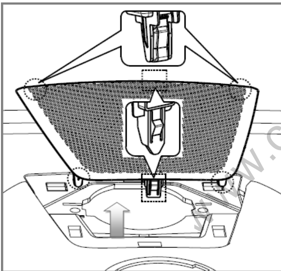
图 1.5.20 中央扬声器罩装配状态
