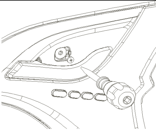
图1.9.6 内扣手螺钉
