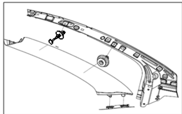
图 1.7.2 A 柱上护板的拆卸
