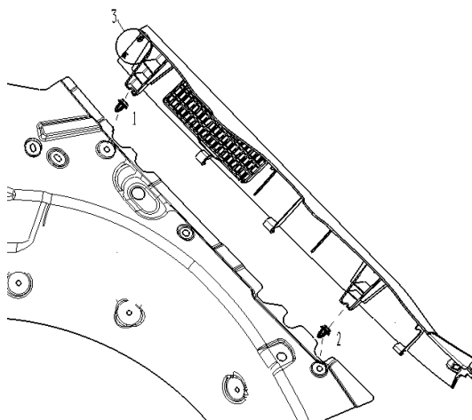
图 1.7.10 C 柱下护板拆卸
