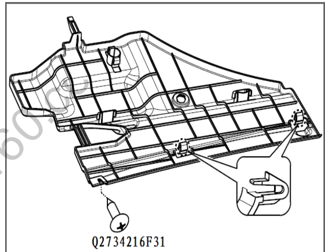
图 1.5.3 仪表板右下隔音板组件
