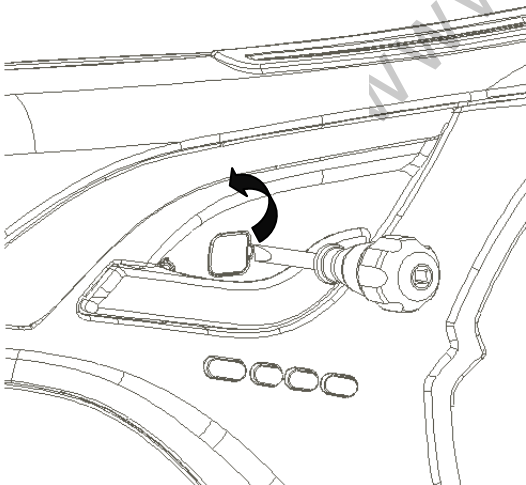
图1.9.2 内扣手盖板
