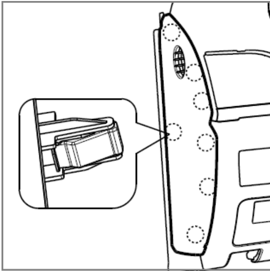
图 1.5.8 仪表板左端护板装配状态
