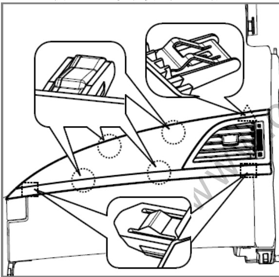
图 1.5.11 仪表板右风口总成
