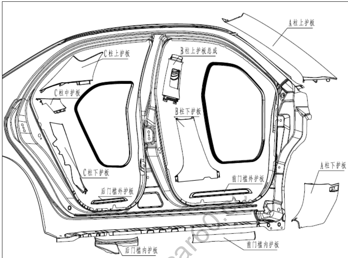
图 1.7.1 侧围系统
