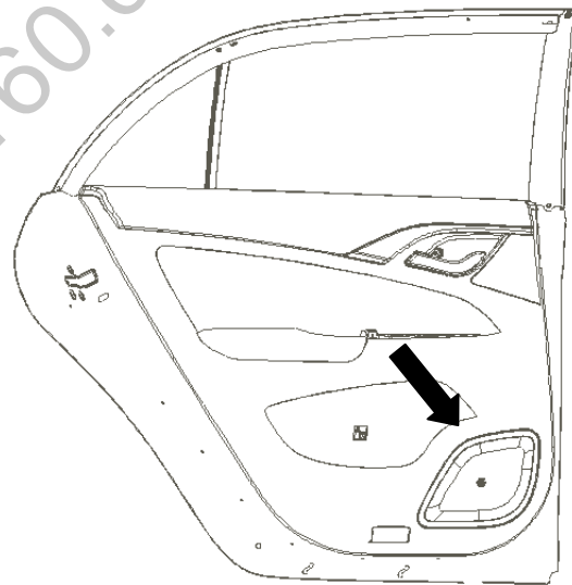
图1.9.19 门护板拆卸
