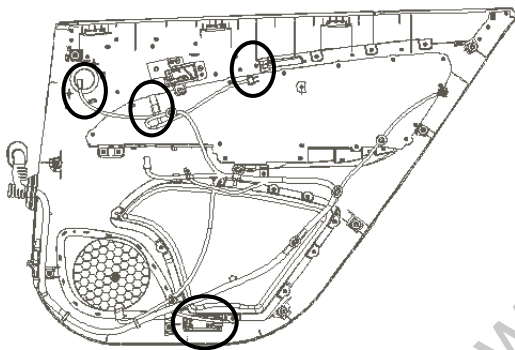
图1.9.22 线束拆卸
