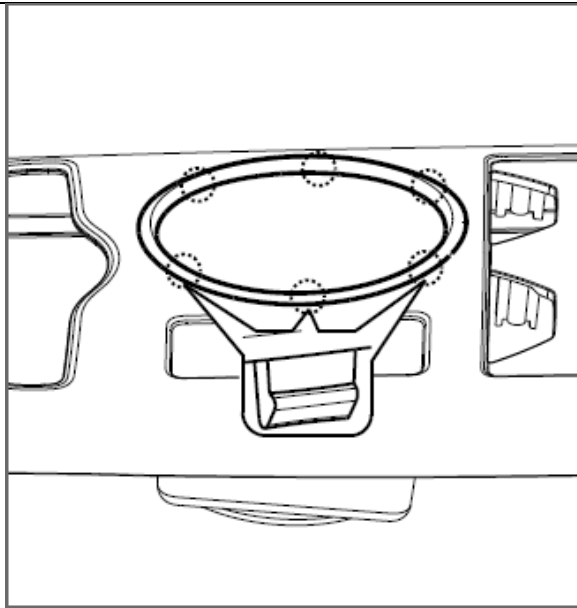
图 1.6.6 前杯托装饰圈的拆卸
