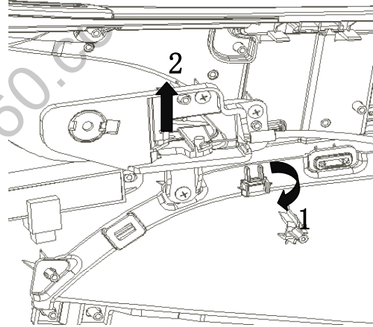
图1.9.9 内开拉锁拆卸
