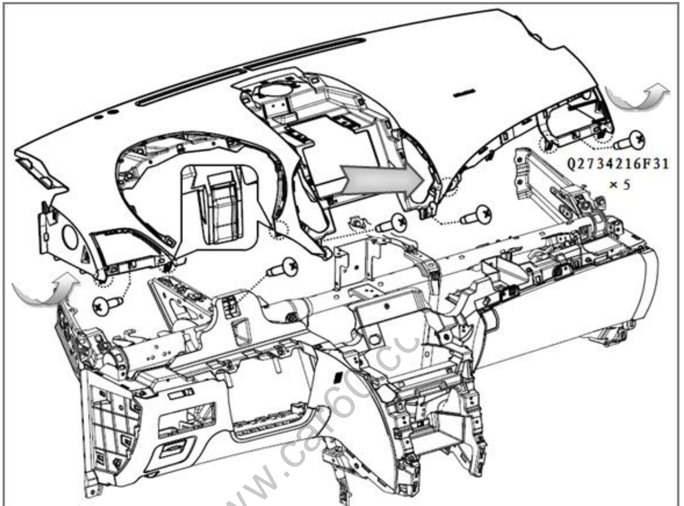
图 1.5.22 仪表板上本体拆卸示意图
