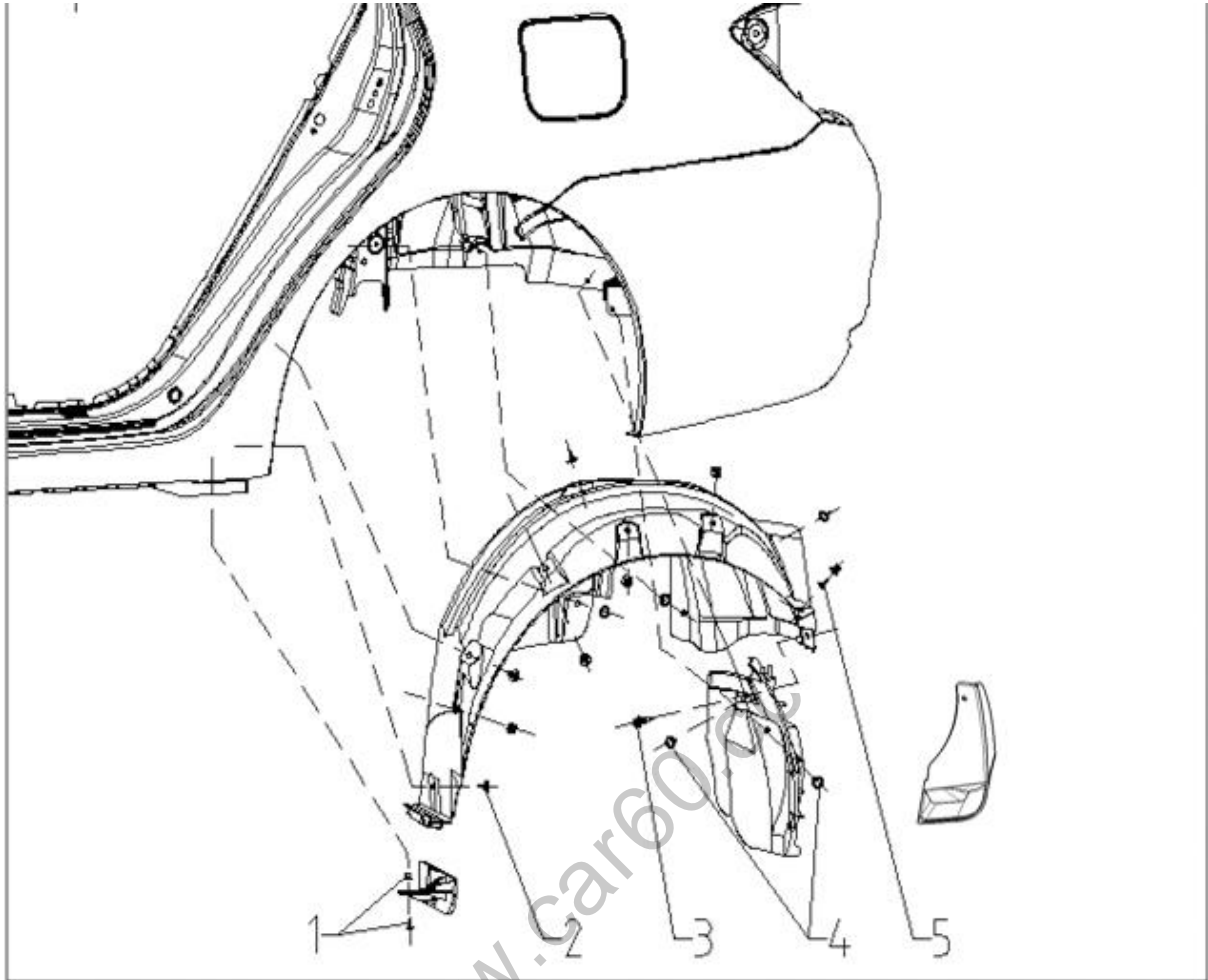
图 1.3.2 后轮挡泥板的拆卸/安装
