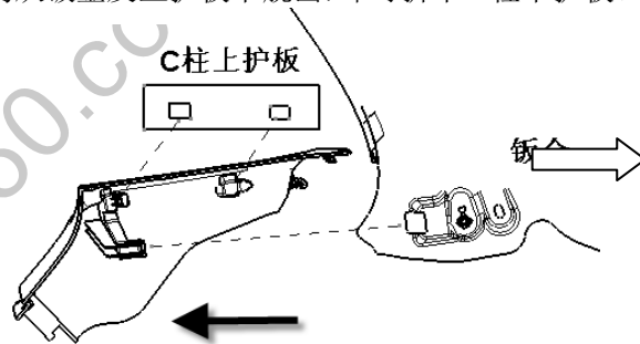
图 1.7.11 C 柱中护板拆卸
