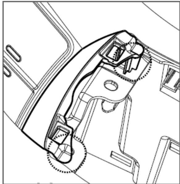
图1.6.8 换挡盖板支撑板的拆卸
