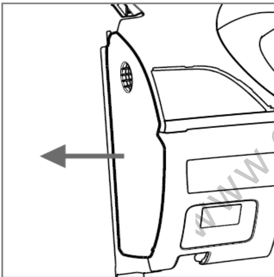
图 1.5.9 仪表板左端护板拆卸示意图
