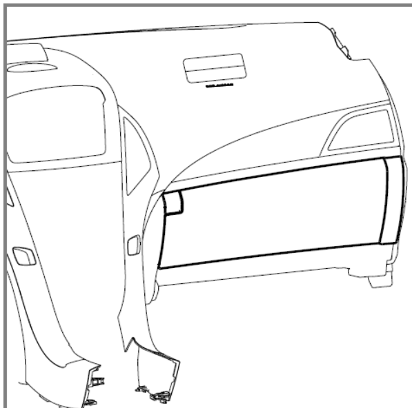
图 1.5.13 杂物箱总成安装位置
