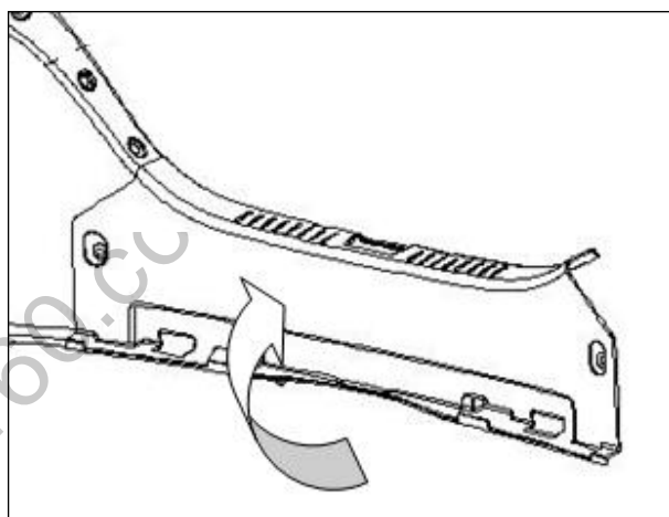
图 1.8.6 后围踏板拆卸示意图
