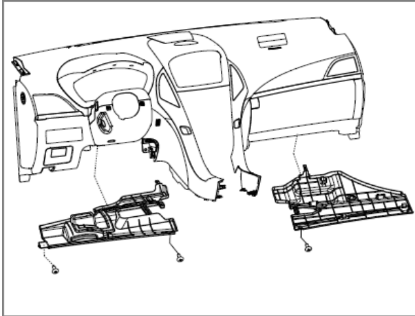
图 1.5.2 隔音板安装位置示意图
