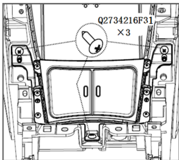
图 1.6.9 前烟灰盒总成的拆卸
