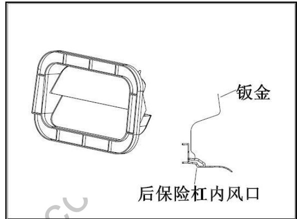
图 1.2.4 保险杠内风口的拆卸
