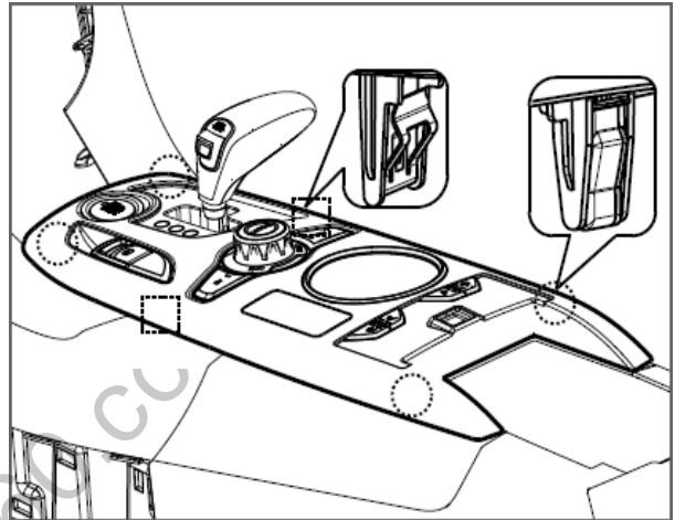
图 1.6.5 换挡操纵机构盖板组件的拆卸
