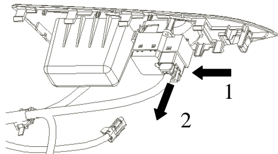
图1.9.15 窗控面板接插件
