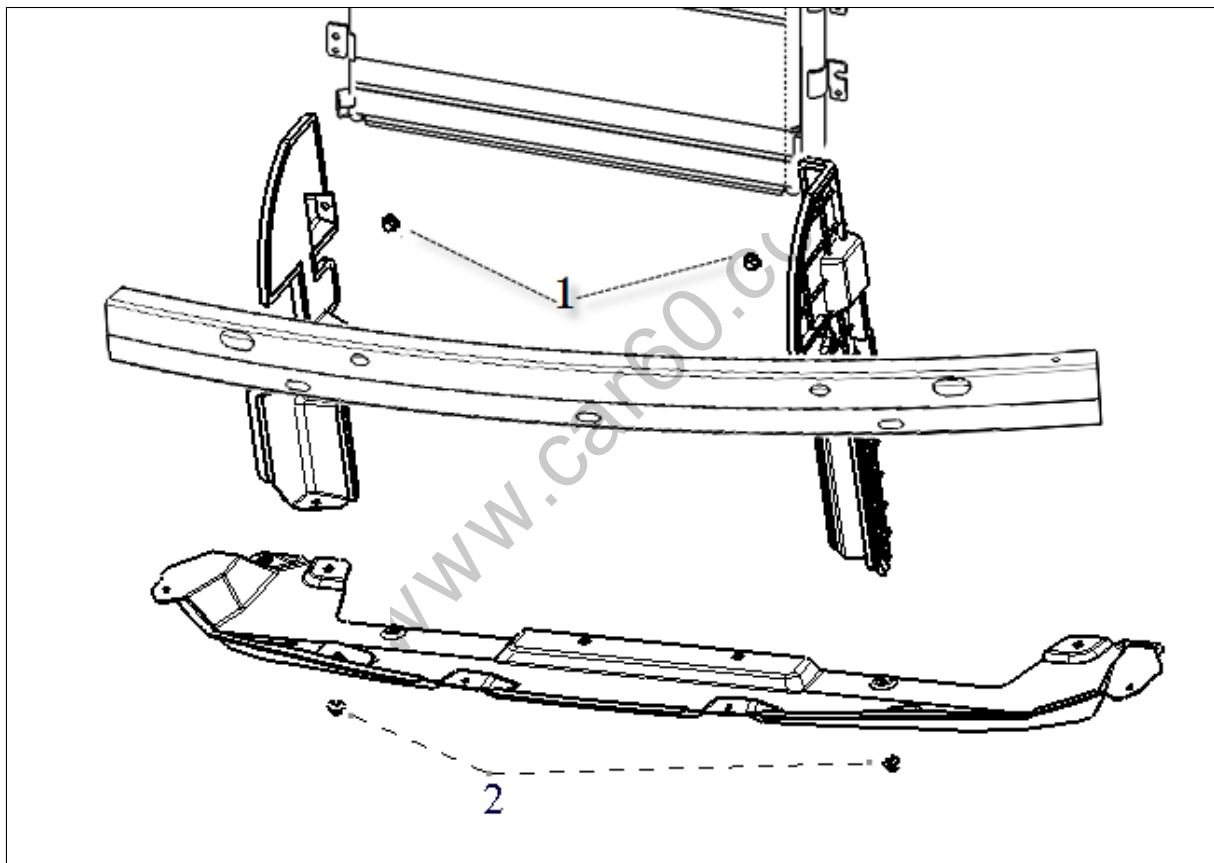
图 1.3.4 导流板的拆卸/安装
