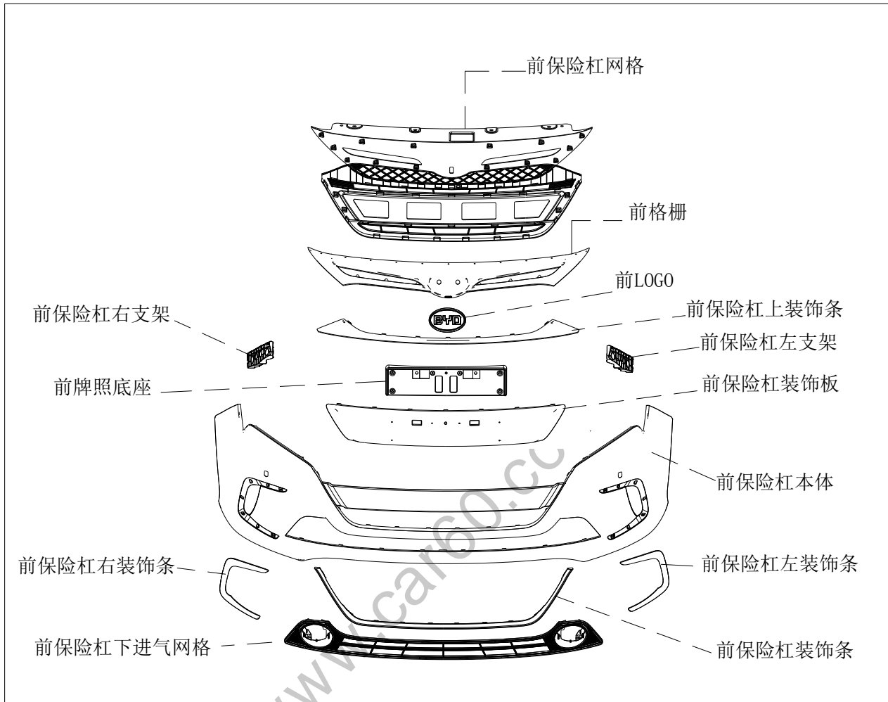
图1.1.1 前保险杠系统组件
