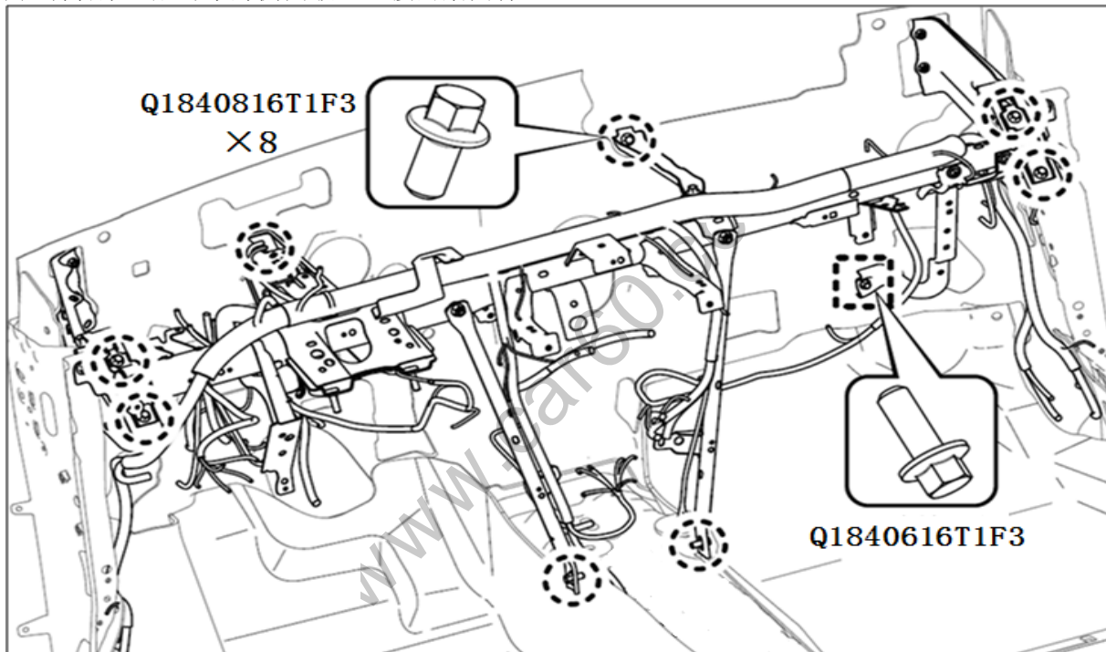
图 1.5.24 管梁总成
