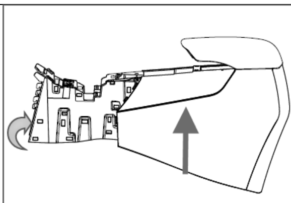
图 1.6.15 副仪表板本体的拆卸
