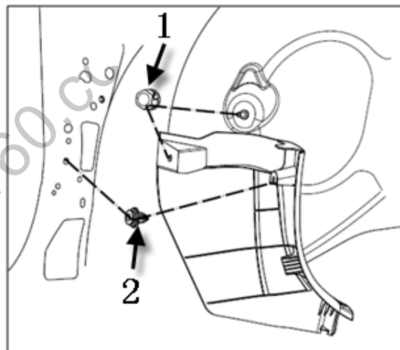
图 1.7.7 A 柱下护板拆卸
