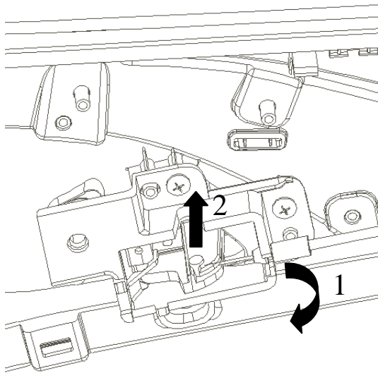
图1.9.20 内开拉锁拆卸
