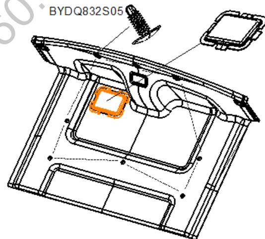
图 1.15.3 行李箱检修口盖板安装结构图
