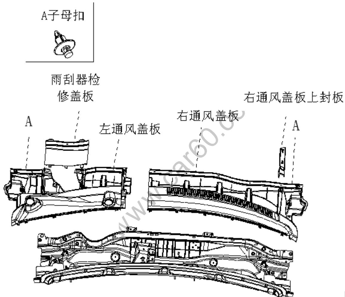
图 1.4.1 通风盖板的拆卸/安装
